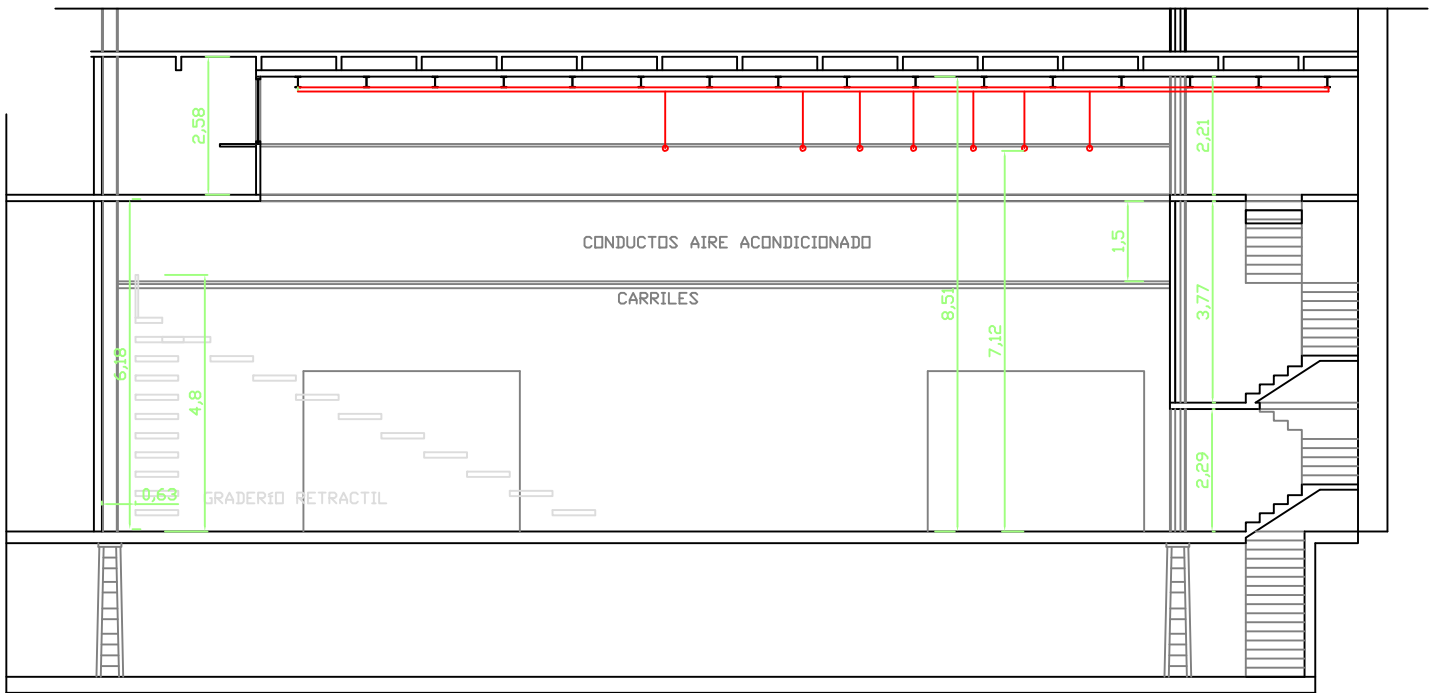
SECCIÓN
